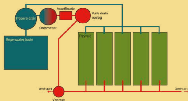
FIGUUR 1 Schema first flush-proefopstelling
